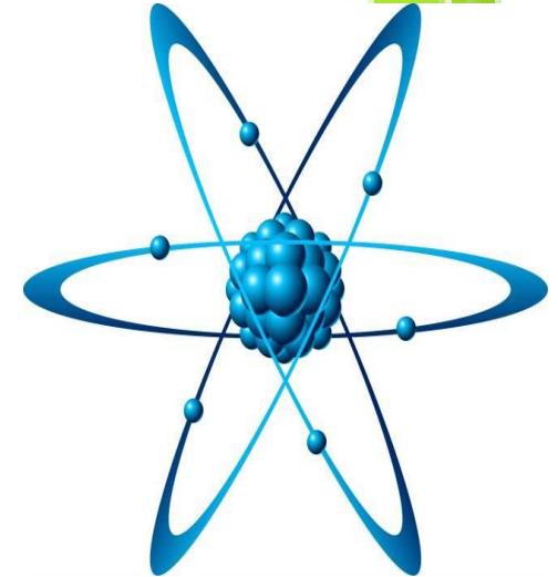
Đêmôcrit
